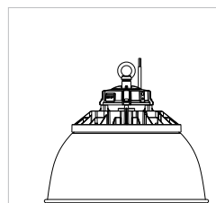
Shade Reflector Aluminium // Schirm Reflektor Aluminium
